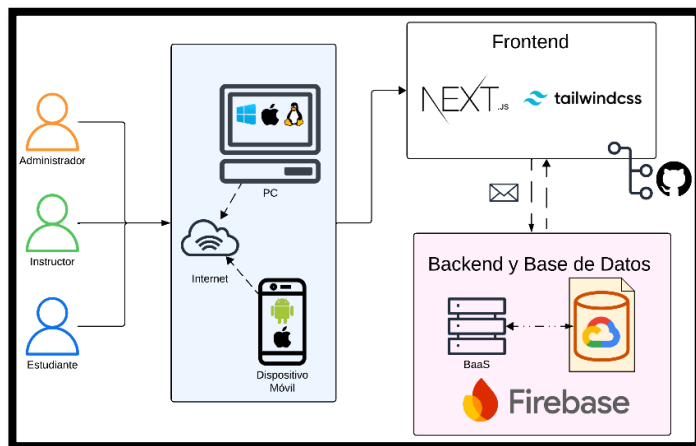
Ilustración 2: Arquitectura Utilizada en el Sistema
