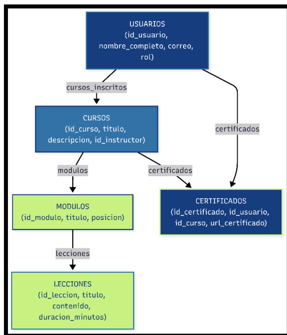
Ilustración 3: Diagrama de Colecciones de la Base de Datos No SQL
