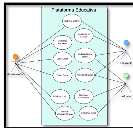
Ilustración 1: Diagrama de Casos de Uso
